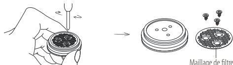
Maillage de filtre
