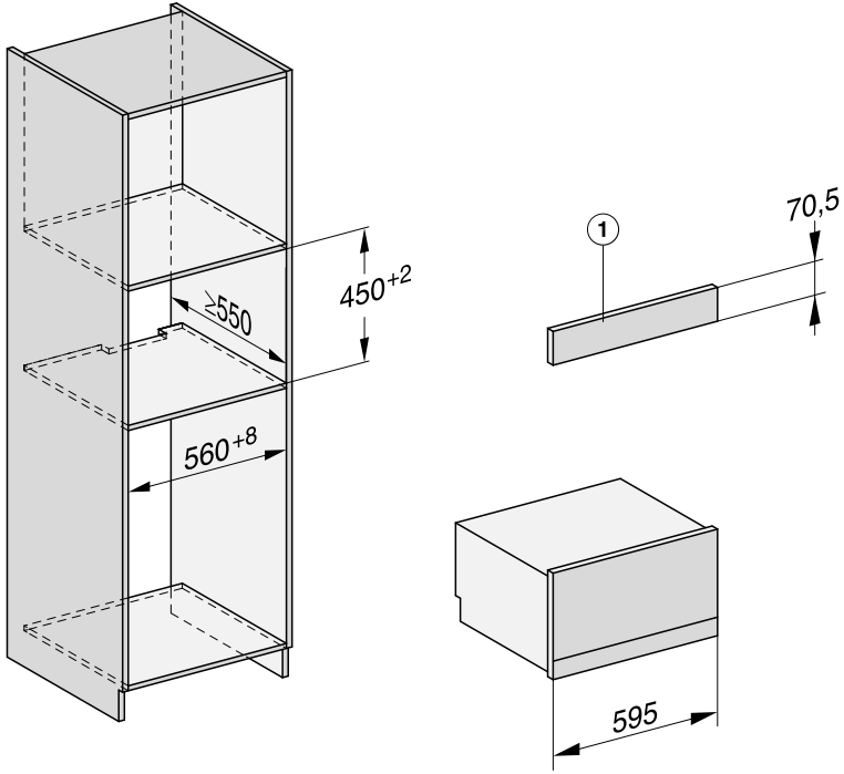
① Opvulpaneel AB 45-7 L
