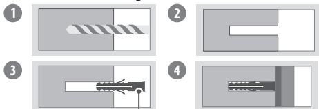
Verankering voor muurbeugel
