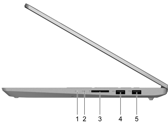
Figure 8. IdeaPad 5 (15", 05) et IdeaPad Slim 5 (15", 05) - vue du côté droit
