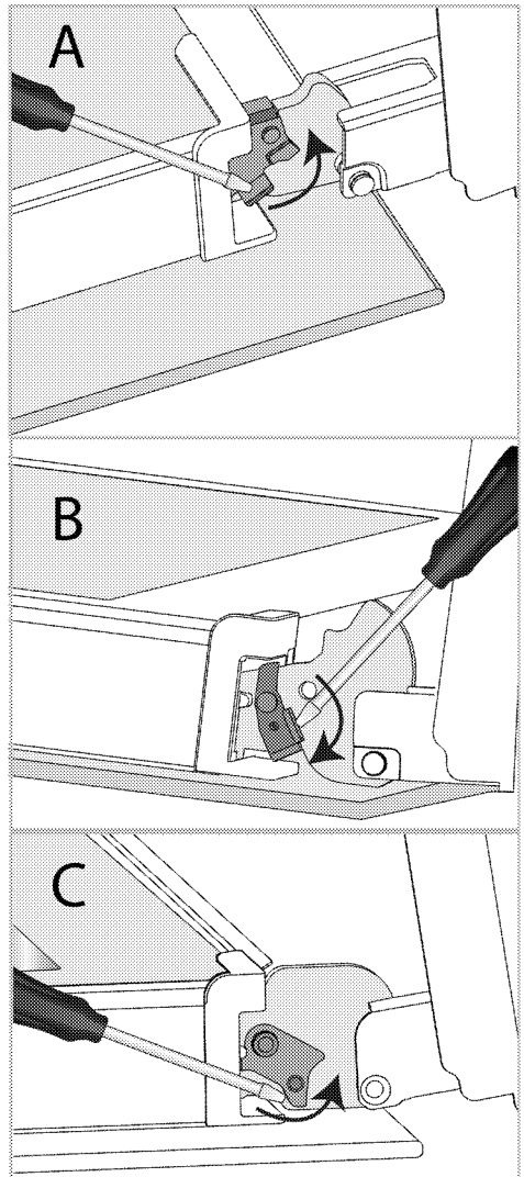
Scharniergevendeling - gesloten positie
