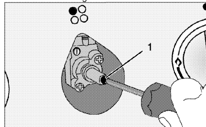
1 Stelschroef gasdebiet
