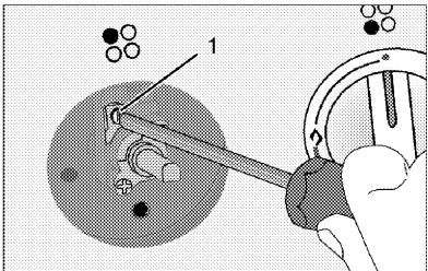
1 Gasdurchfluss-Einstellschraube
