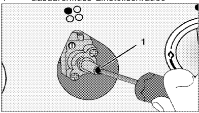
1 Gasdurchfluss-Einstellschraube
