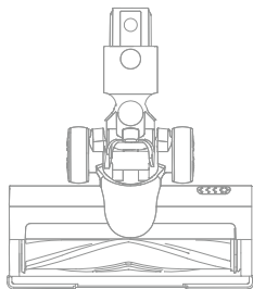
Elektrischer Staubsaugerkopf
