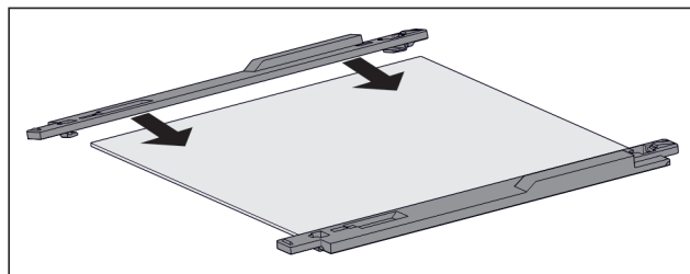
Fig. 44 Tablette en verre avec pièces de retenue
