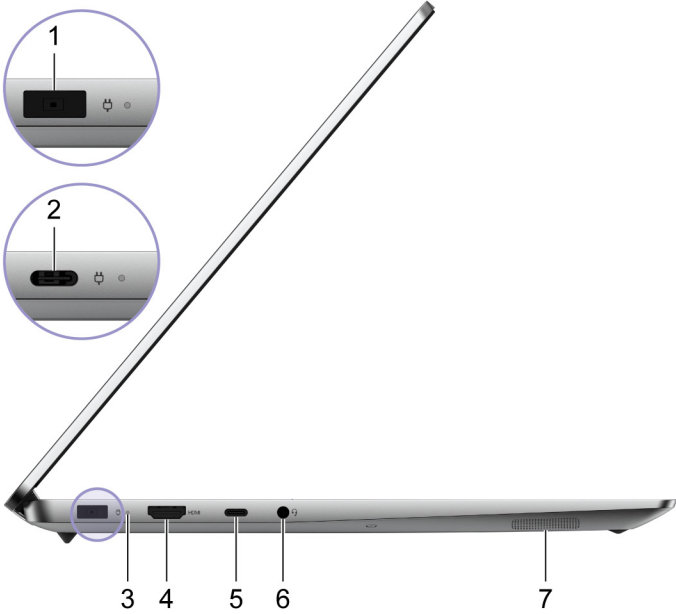
Figure 4. Vue du côté gauche—IdeaPad 5 Pro 16ACH6
