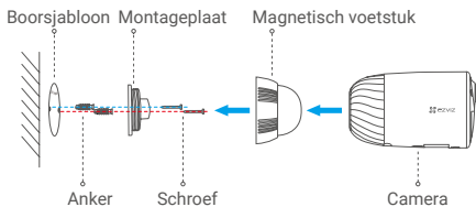
Afb. 1 Montage met magnetische basis
