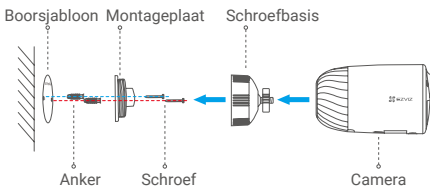
Afb. 2 Montage met schroefbasis
